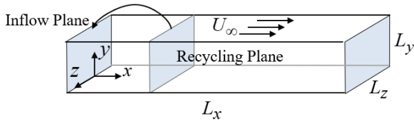
شکل ۱ - شماتیک مفهومی از مدل مرز ورودی لاند
