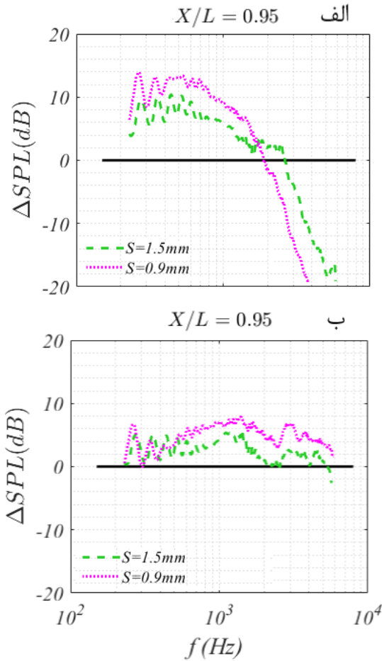
شکل ۱۴ - اختلاف سطح نوپز پیش‌بینی شده با مدل تحلیلی راجر-امیت [۱] در فاصله عمودی y' = 1 \text{ m} از سطح مدل با دو طول مختلف، (الف) L = 0.27 \text{ m} ، (ب) L = 0.3 \text{ m} .
