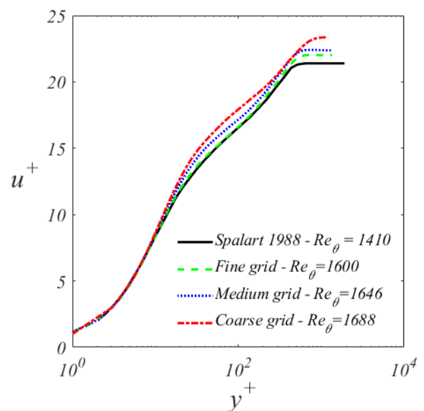
شکل ۴ - پروفیل سرعت متوسط بر حسب فاصله از دیواره در
