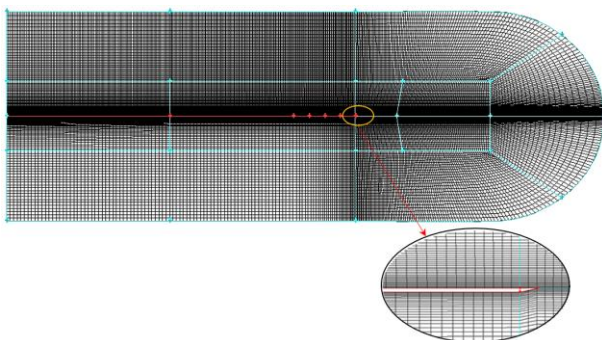
شکل ۳ - بلوک‌بندی سطح جانبی و نمای کلی شبکه محاسباتی
