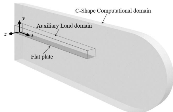
شکل ۲ - میدان حل محاسباتی C شکل
