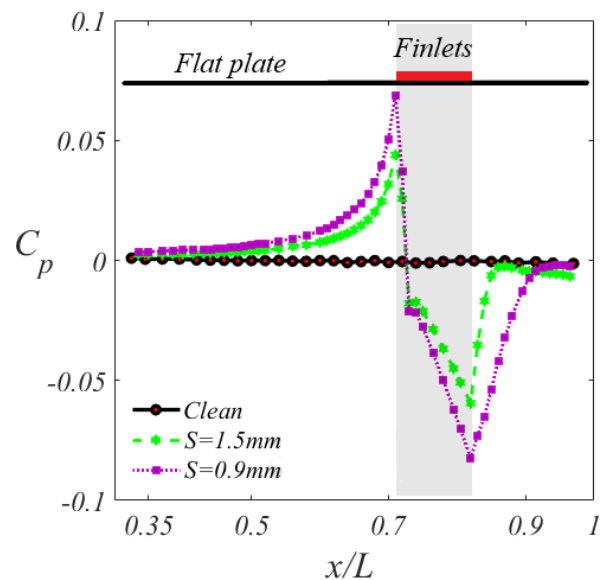
شکل ۸ - توزیع ضریب فشار استاتیک بر روی خط میانه عرضی صفحه تخت مجهز به فینلت‌ها در مقایسه با صفحه تخت مینا در فاصله 98\% \leq x/L \leq 35\% .
