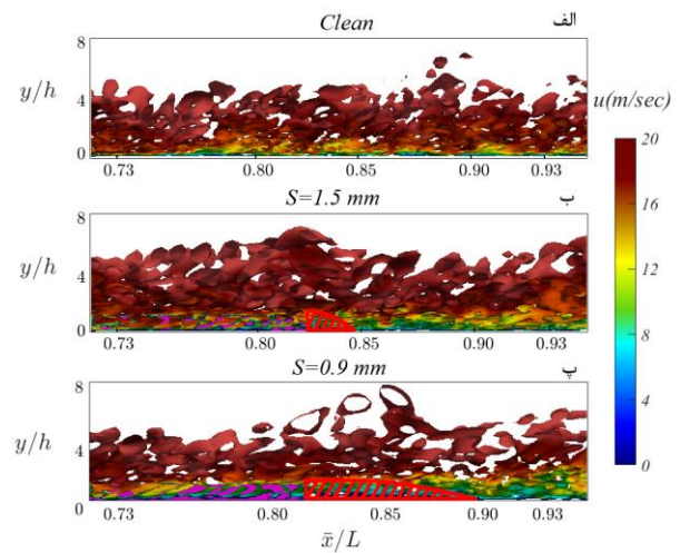
شکل ۱۳ - سطوح همتراز معیار کیو ( Q=1 \times 10^5 )، رنگ آمیزی شده با مقادیر سرعت لحظه‌ای در محدوده 0.71 < x/L < 0.95 . (الف) حالت مبنا، (ب) فاصله عرضی بین فینلت‌ها S = 1.5 \text{ mm} و (پ) فاصله عرضی بین فینلت‌ها S = 0.9 \text{ mm} .
