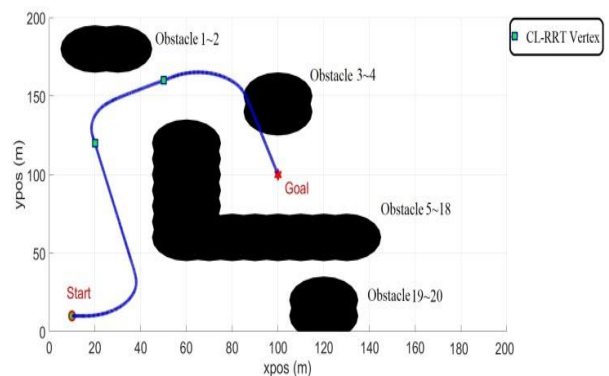
شکل ۱۴- نما از بالای فضای پیکربندی تست شماره دو، به همراه مسیر طراحی شده توسط الگوریتم طراحی مسیر پیشنهادی و نقطه مسیره‌های که با مربعات سبز رنگ نمایش داده شده‌اند.
