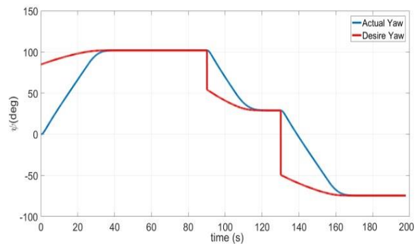
شکل ۱۳- مسیر مطلوب با خط قرمز رنگ و مسیر واقعی ربات با خط آبی رنگ نمایش داده می‌شود.
