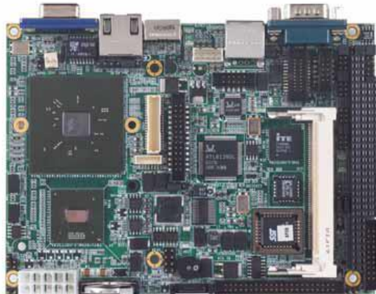
شکل ۳- پردازنده هدف SBC84710 مورد استفاده در تست پردازنده در حلقه در محیط xPC-Target نرم افزار متلب
