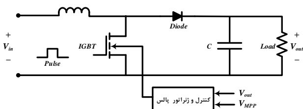
شکل ۶- شماتیک یک مبدل بوست [۲۹]
