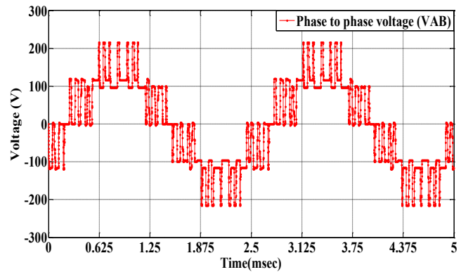
شکل ۱۸- ولتاژ خروجی مبدل DC/AC بدون فیلترینگ، ولتاژ بین
