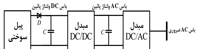
شکل ۵- بلوک دیاگرام نحوه اتصال پیل سوختی به باس ضروری جریان متناوب ۱۶ هواپیمای C-130
