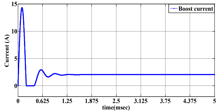
شکل ۱۴- جریان گذرنده از سلف مبدل DC/DC بوست
