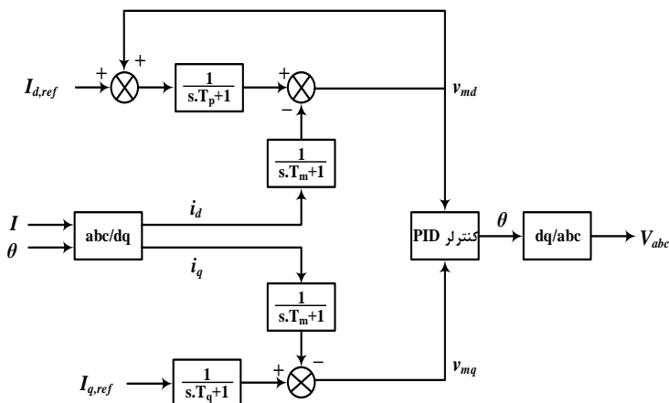
شکل ۱۱- بلوک دیاگرام سیستم کنترلی اینورتر [۳۱]
