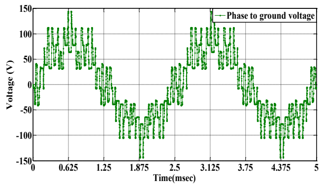
شکل ۱۹- ولتاژ خروجی مبدل DC/AC بدون فیلترینگ، ولتاژ بین فاز و
