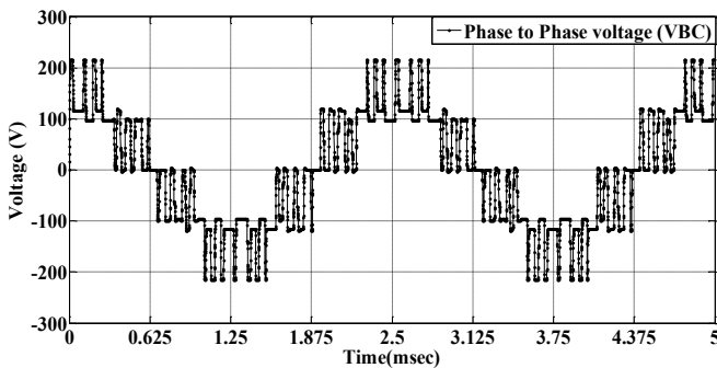
شکل ۱۶- ولتاژ خروجی مبدل DC/AC بدون فیلترینگ، ولتاژ بین فازهای B و C
