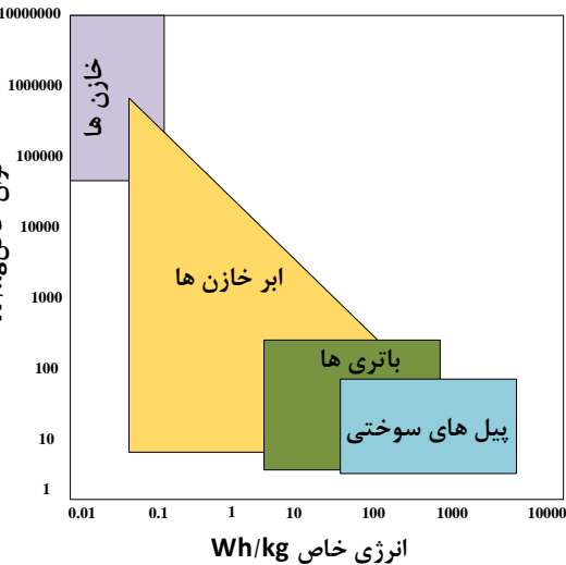
شکل ۱- مقایسه چگالی توان و انرژی پیل های سوختی با باتری و خازن [۲۱]
