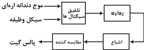
شکل ۹- شماتیک مدار داخلی تولیدکننده ی پالس [۳۰]
